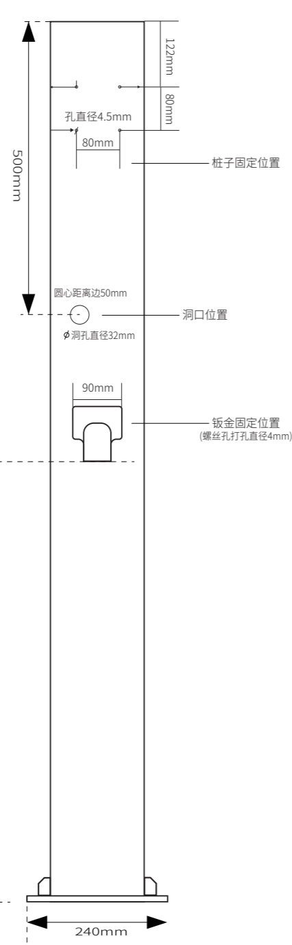
正视图
