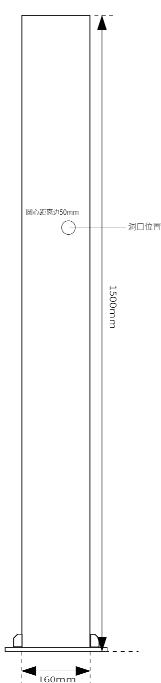
背视图
