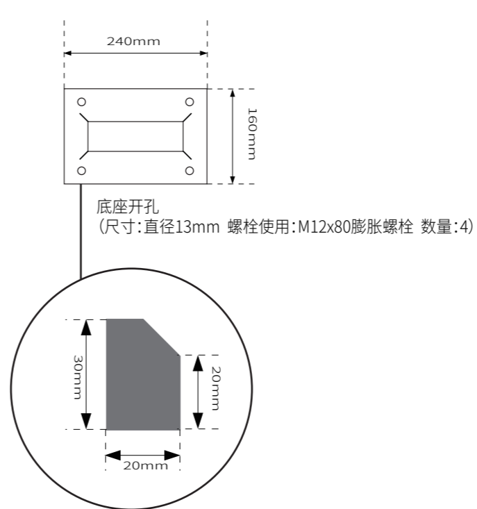
顶视图
